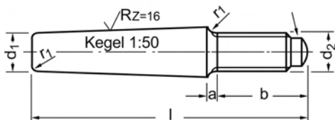
Ansatzkuppe nach DIN 78
