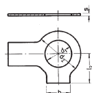
DIN 463
