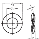
DIN 137 B
