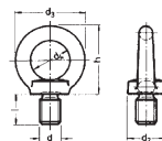
DIN 580
