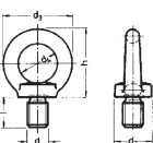
DIN 580
