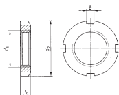
DIN 981
