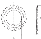
DIN 5406
