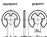
DIN 7993 B
